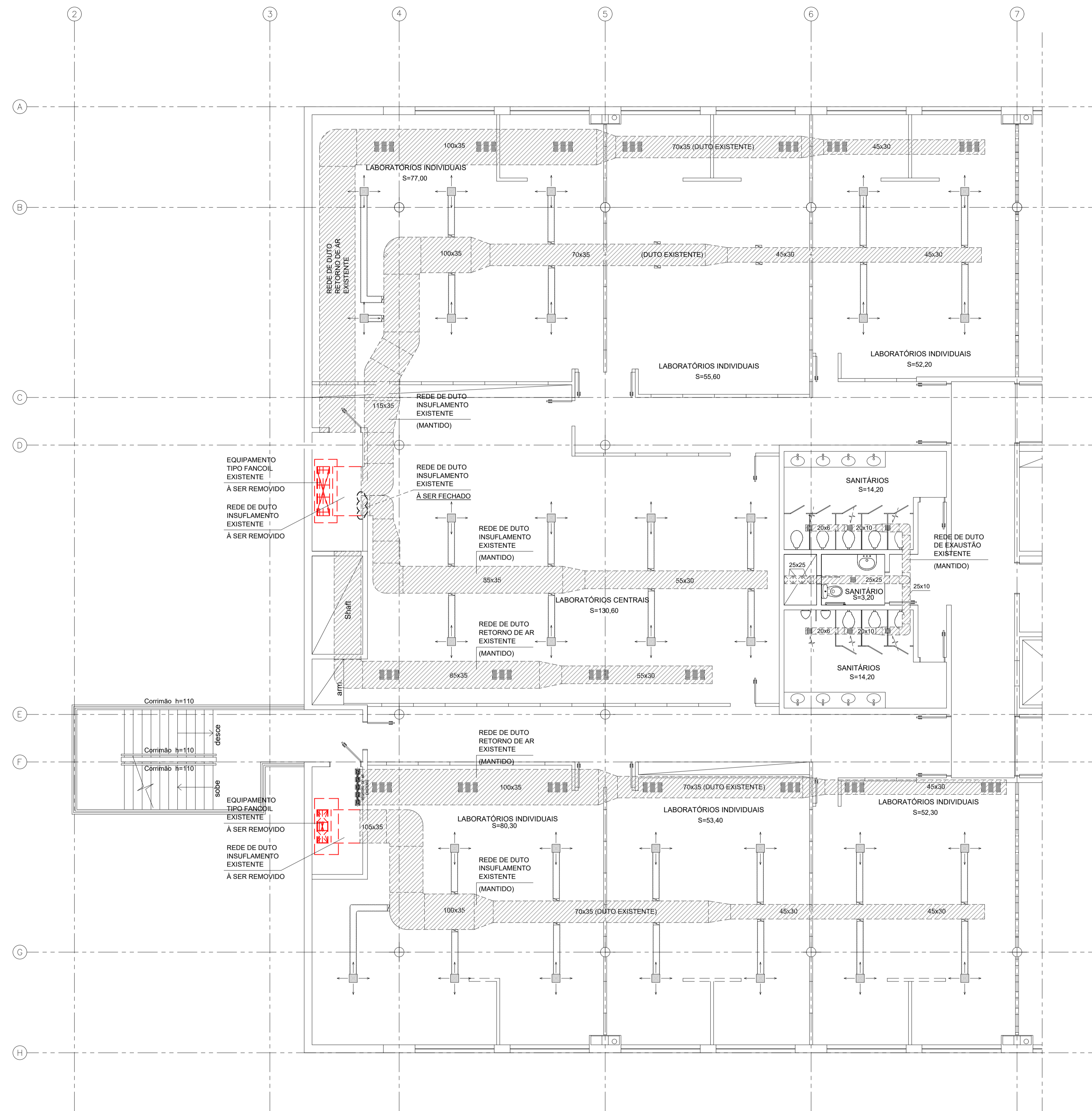
PLANTA DO 2º PAVIMENTO / PARCIAL - INSTALAÇÃO EXISTENTE ESCALA - 1:75
